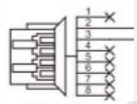
TMT 2*4
