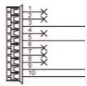
MOLEX 51004-10P
